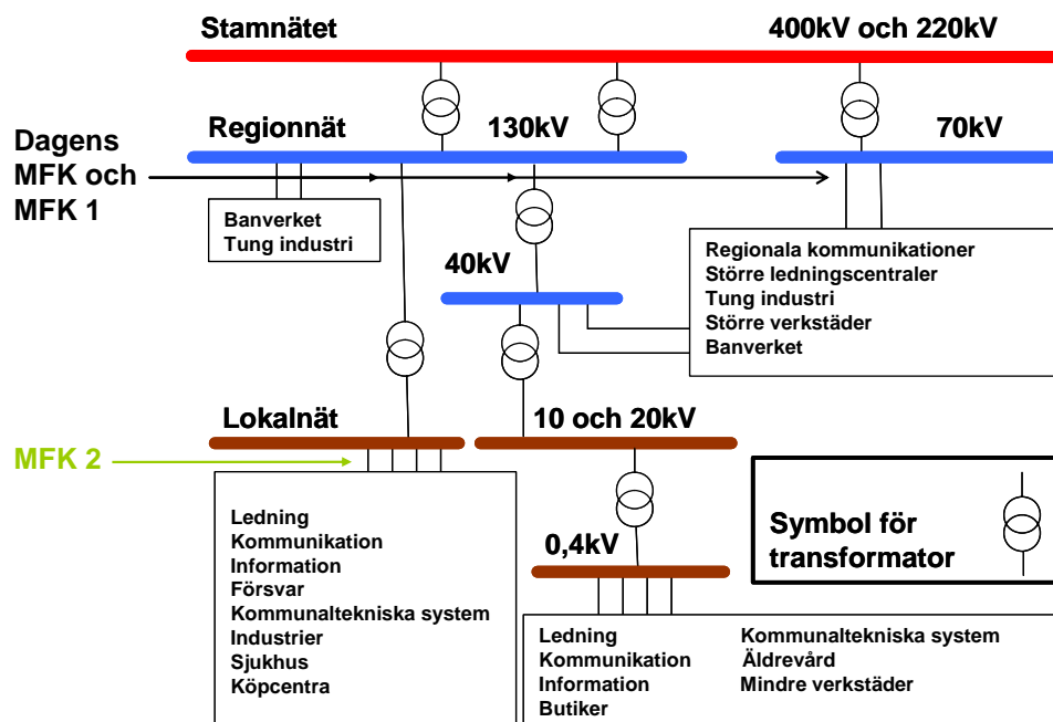
Figur 4.1 Nätets struktur, och olika typer av elanvändares lokalisering på elnäten
