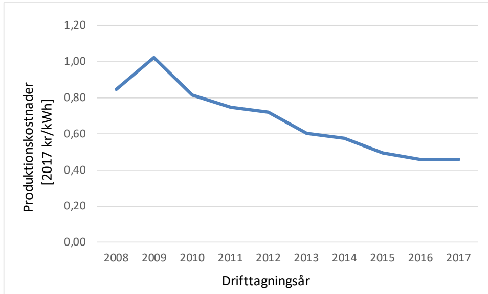
Figur 7. Utvecklingen av produktionskostnaderna för vindkraft under perioden 2008–2017, SEK 2017/kWh.
