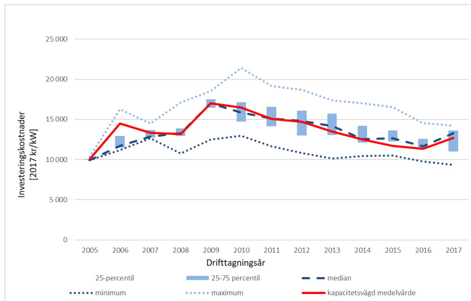
Figur 4 - Investeringskostnader för vindkraftsprojekt som tagits i drift perioden 2005–2017, SEK 2017 per kW. Omräknade till SEK 2017 med Världsbankens BNP-omräkningsfaktor.
